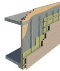
Fachada ventilada
