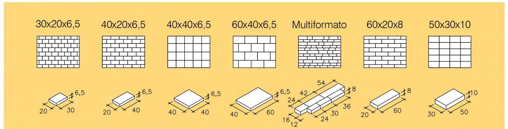
Fig. superior: Despiece en planta de un pavimento de 2,00 x 1,50 m ejecutado con el formato correspondiente. Fig. inferior: Vista en axonometría de cada formato de pavimento.
