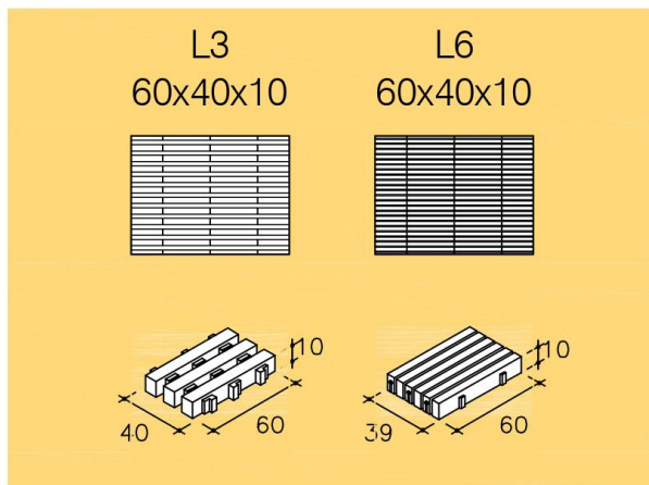
Fig. superior: Despiece en planta de un pavimento de 2,00 x 1,50 m ejecutado con el formato correspondiente. Fig. inferior: Vista en axonometría de cada formato de pavimento.
